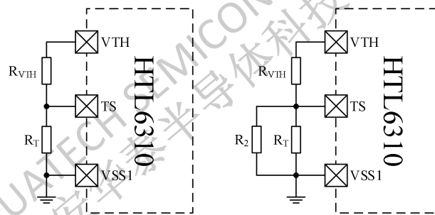
图 13 (a) R_{VTH}+R_T 方式
