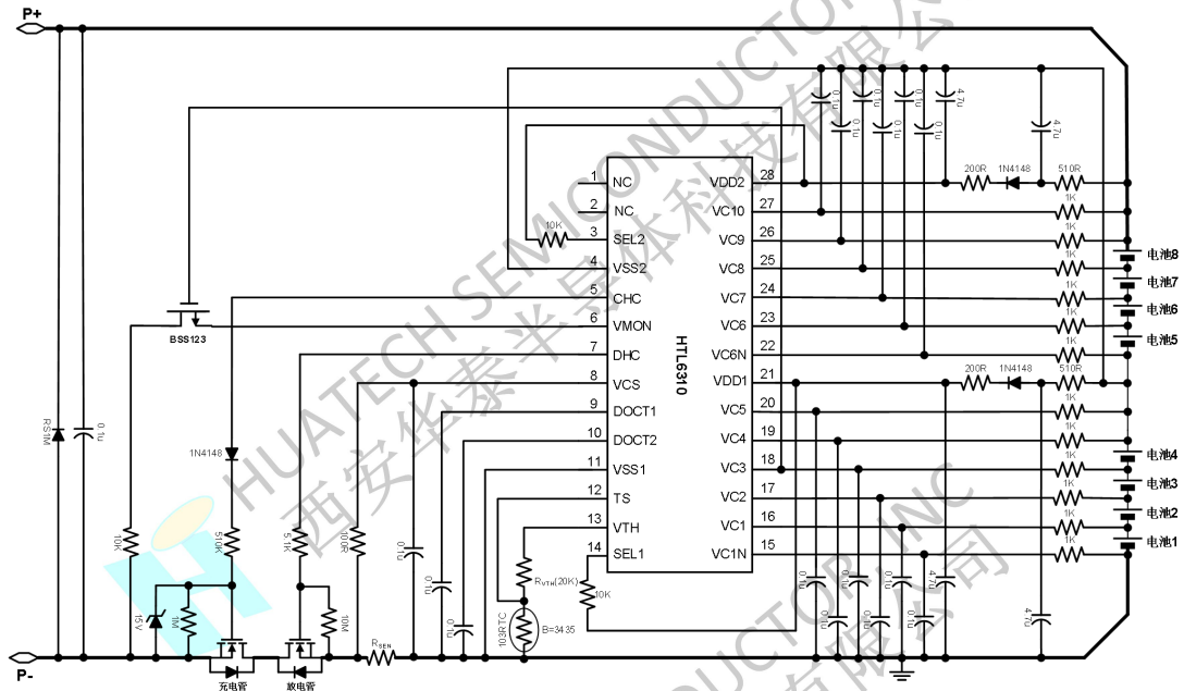
图 4 8 节电池包的 N 型充电管和 N 型放电管的同口典型应用电路图
