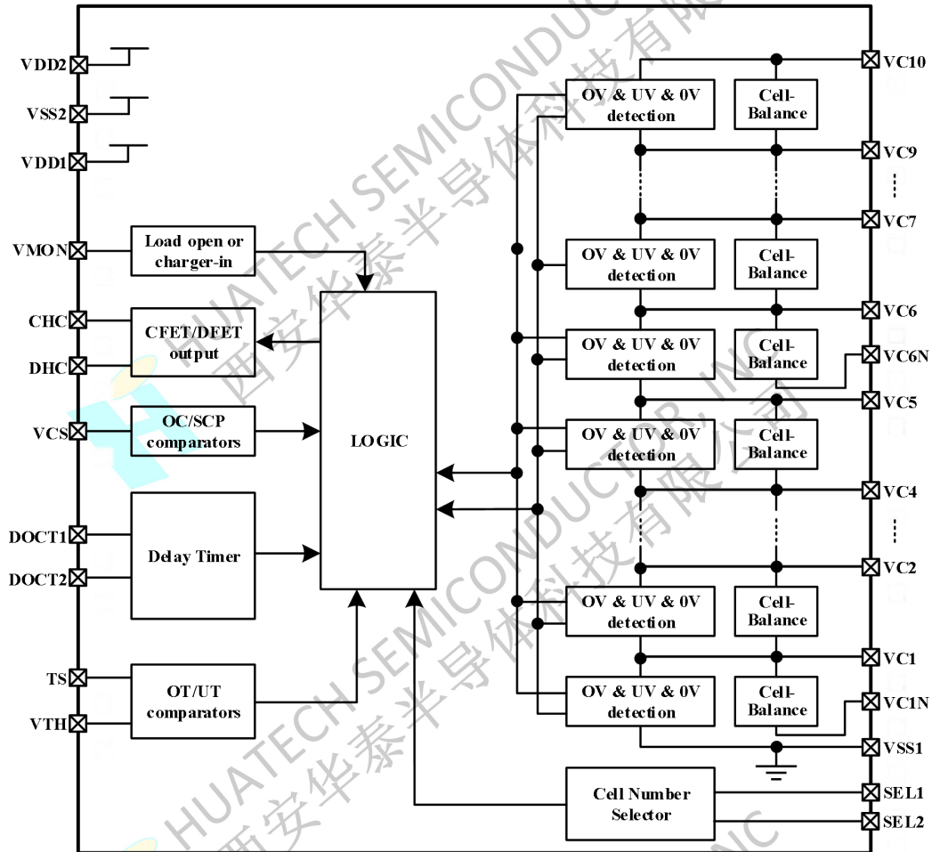
图 8 功能框图
