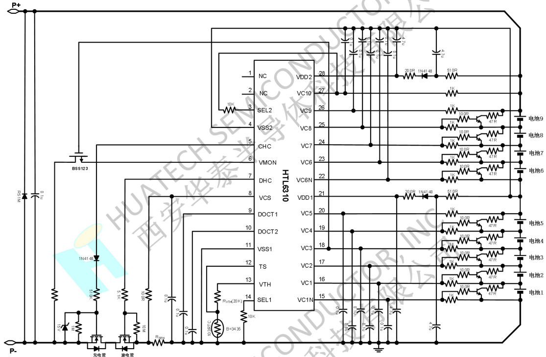
图 6 9 节电池包外部扩展均衡的 N 型充电管和 N 型放电管的同口典型应用电路图
